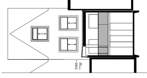
doorsnede E-E
